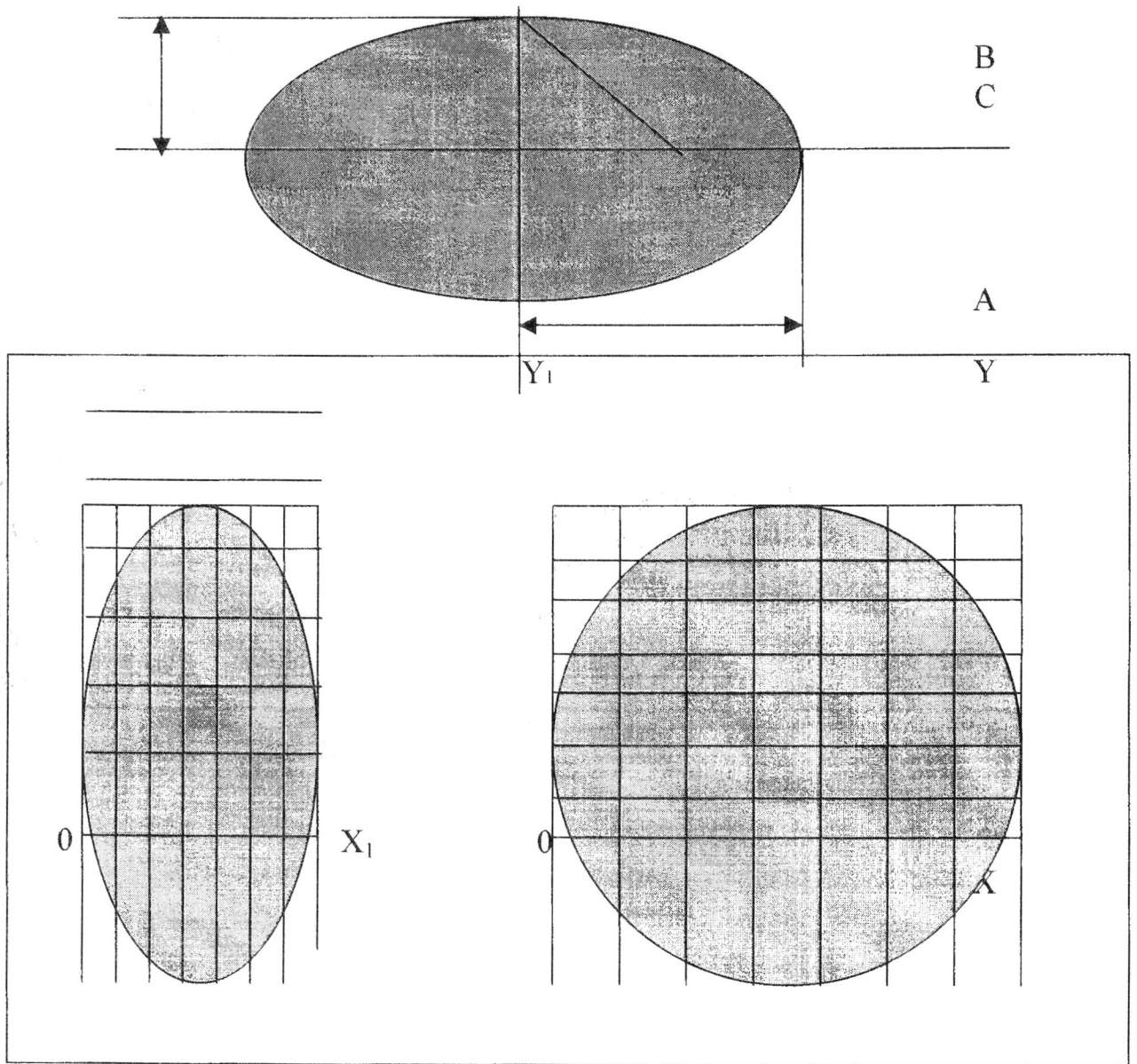
شكل 3- تطبيق المبدأ الذي اعتمده (Thompson) في اشتقاق الشكل المثالي للمبنى [الباحثان].
