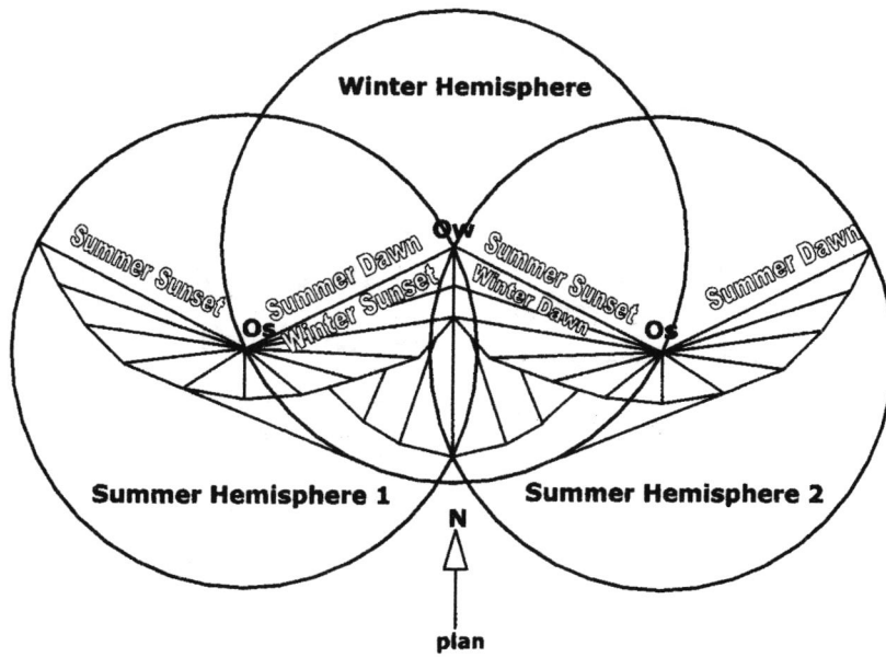
شكا 2- الشكا الذي خرجت به دراسة Knowles، بأعتماد حركة الشمس كأساس، لتولد الشكا [6]
