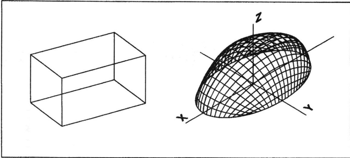
شكل 5- الشكل المثالي (thermal hemisphere) مقارنة مع الشكل بمفهوم (thermal cube) الذي خرجت به الدراسات السابقة [الباحثان بواسطة برنامج AutoCAD2000]
