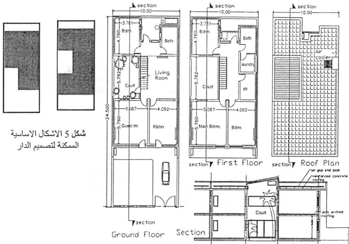
الشكل 6 الخرائط الاساسية للدار البني المقترح وتشمل من اليسار خارطة الطابق الارضي والاول والسطح ومقطع في الدار يمر بالفناء في الاسفل
