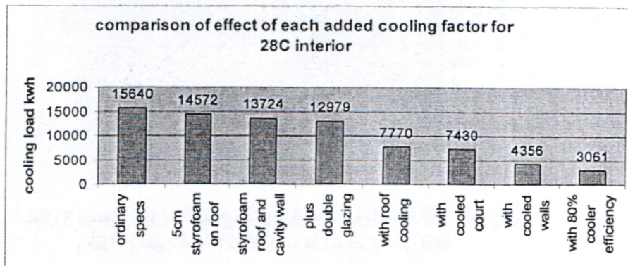
شكل 12 رسم توضيحي لطاقة التبريد الكلية للدار بعد اضافة كل حل تبريدي.
