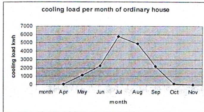
شكل 14 حمل التبريد لكل شهر للدار الاعتيادية المبردة.
