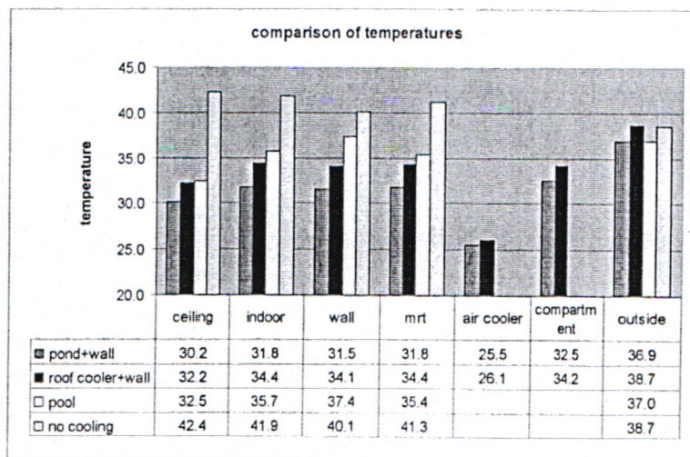
شكل 3 مختصر نتائج كافة تجارب التبريد التي جرت على غرفة الاختبار
