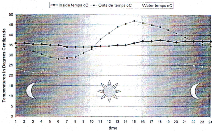
شكل 2 درجات الحرارة داخل وخارج غرفة الاختبار بعد استخدام الحوض السطحي
