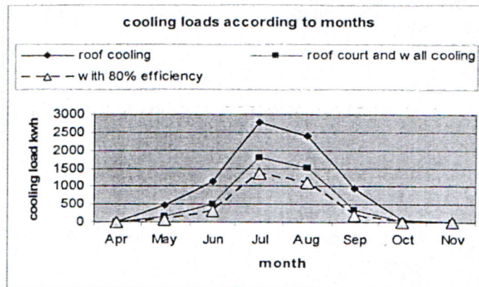
شكل 15 حمل التبريد الشهري للتبريد السطحي وباضافة تبريد الجدران والفناء واخيرا لزيادة كفاءة المبردة التبخرية الى 80%.
