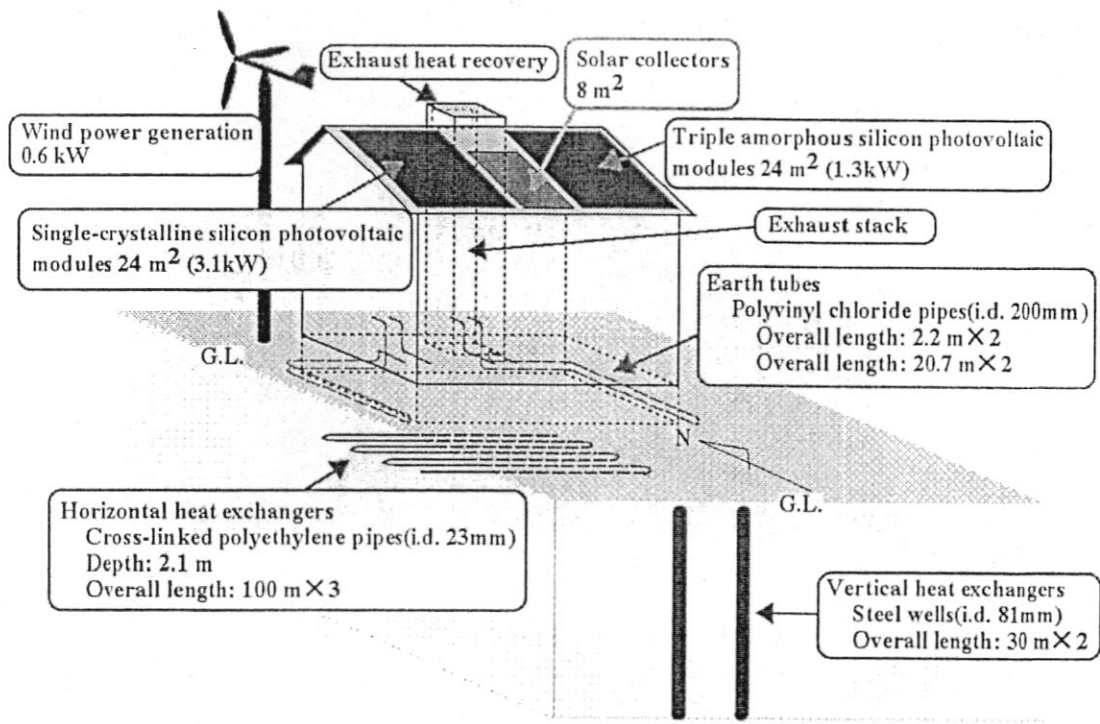
شكل 4 رسم توضيحي للمعالجات البنائية في دار هوكانيدو [2]
