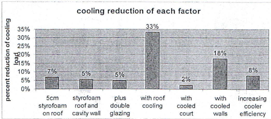
شكل 13 التوفير في الطاقة لكل حل بيئي بصورة منفردة مقارنة مع الدار التقليدي.
