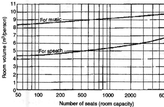
شكل ١-١٠ الحدود الدنيا لاحجام القاعات
