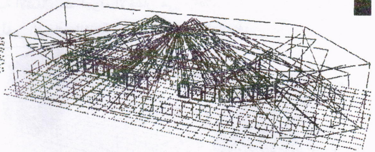
شكل ١٣-٣ توزيع الطاقة الصوتية في القاعة بعد اضافة القواطع المنحنية واللوحات المعروضة
