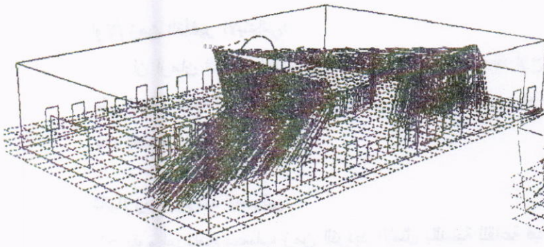
شكل ٢٣-٣ تعزيز الطاقة الصوتية بواسطة العواكس
