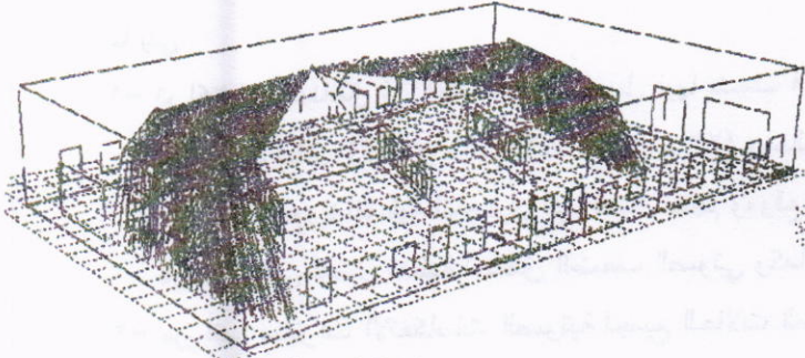
شكل ٢٠-٣ تعزيز الطاقة الصوتية بواسطة العواكس
