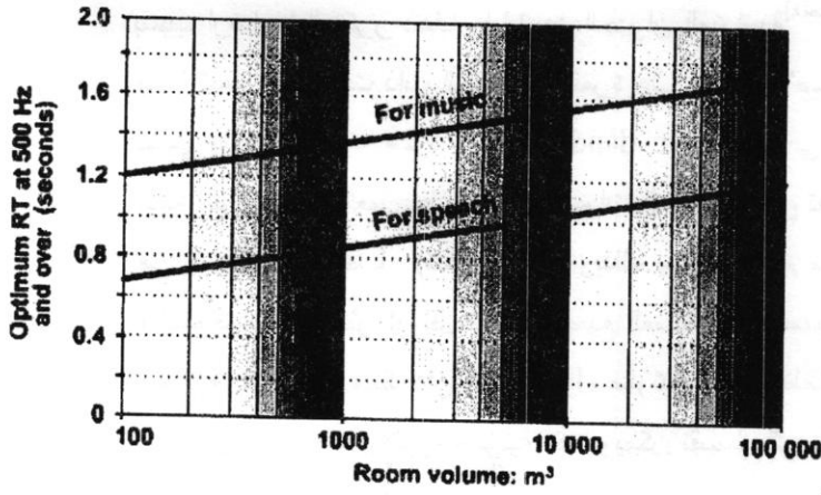
شكل ١١-١ علاقة زمن التردد الصوتي بحجم الفضاء
