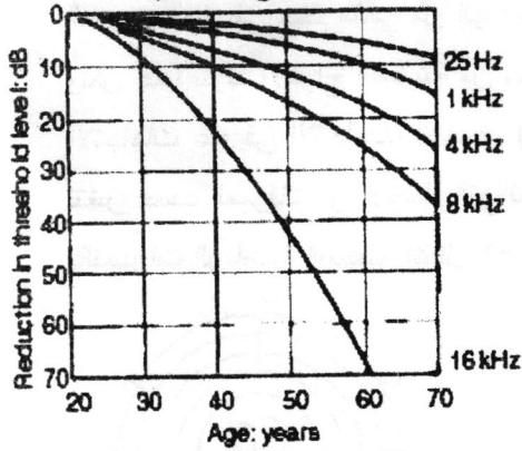
شكل ٧-١ علاقة العمر بحساسية الاذن
