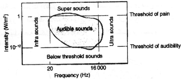
شكل ٦-١ المدى الصوتي المسموع
