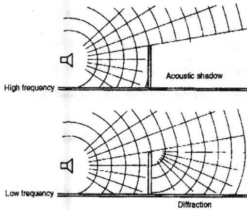
شكل ١٣-١ ظاهرة الحيود الصوتي
