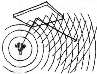
شكل (٤-١) تشكيل الحقل الصوتي
