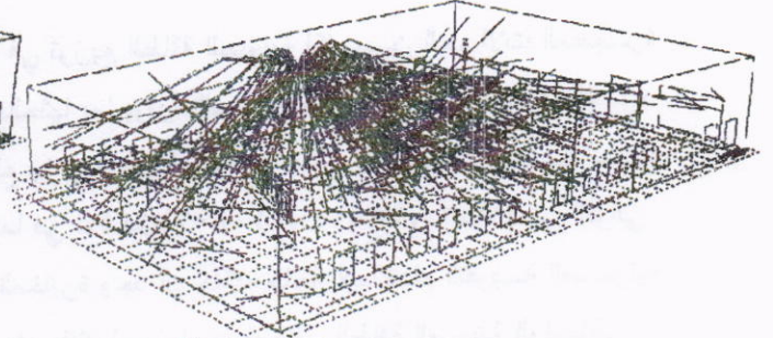
شكل ١٩-٣ توزيع الطاقة الصوتية في القاعة بعد اضافة القواطع واللوحات المعروضة
